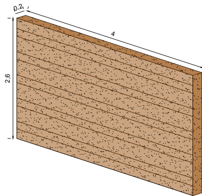
ΑΞΟΝΟΜΕΤΡΙΚΟ ΤΟΙΧΩΝ RAMMED EARTH W.C.
