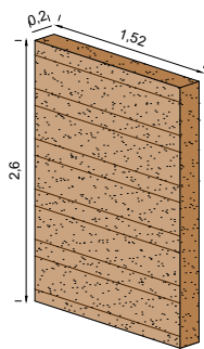
ΑΞΟΝΟΜΕΤΡΙΚΟ ΤΟΙΧΩΝ RAMMED EARTH W.C.
