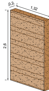
ΑΞΟΝΟΜΕΤΡΙΚΟ ΤΟΙΧΩΝ RAMMED EARTH W.C.
